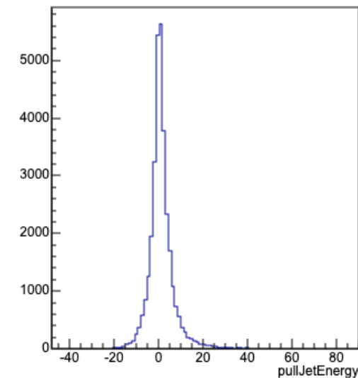
pullJetEnergy
