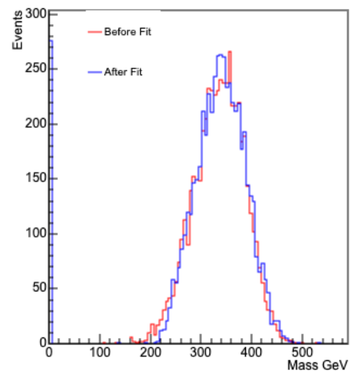
HH Mass
