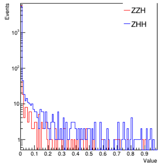
HH Mass
