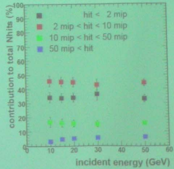
(positron data CERN2006)
