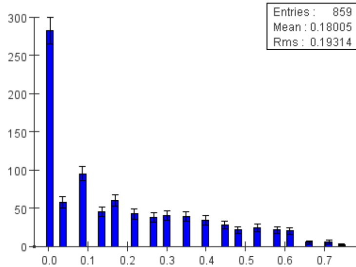
Tr Mip Clus E
