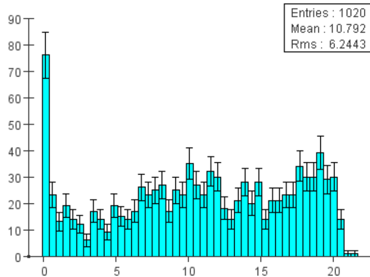
Tr ILSP Clus E
