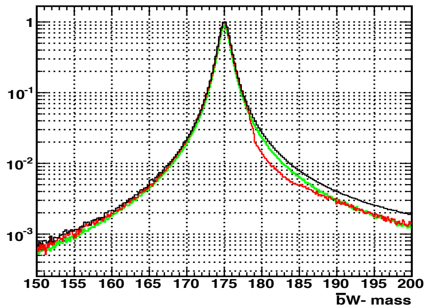
\bar{b}W^- (em-1.0,ep0.0)
