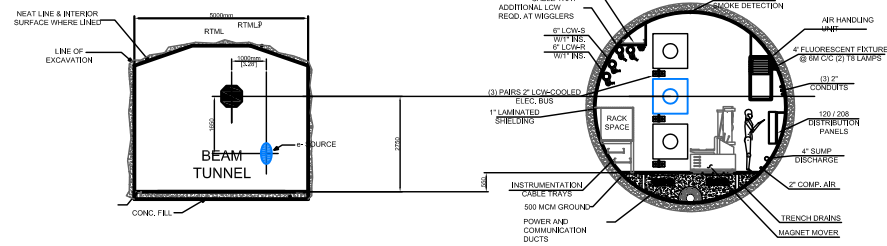
SECTION @ ELTR (H)
