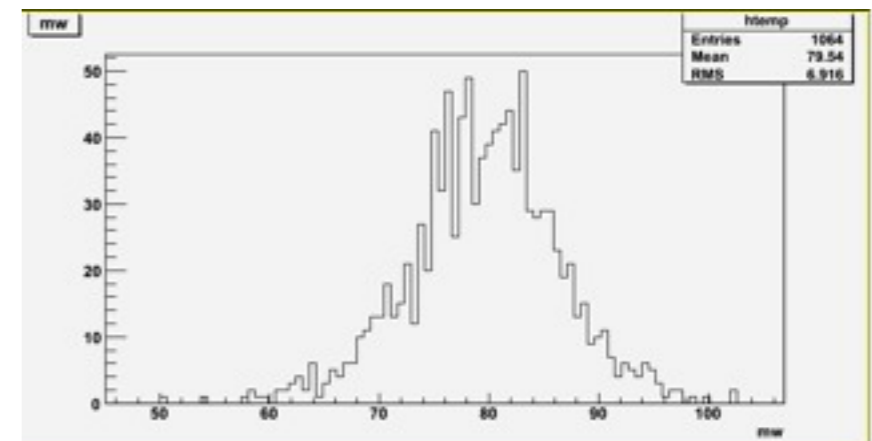
W mass
