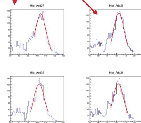
シングルヒットイベントのヒストグラム 横軸はADC値でシングルヒットの電荷量に対応
