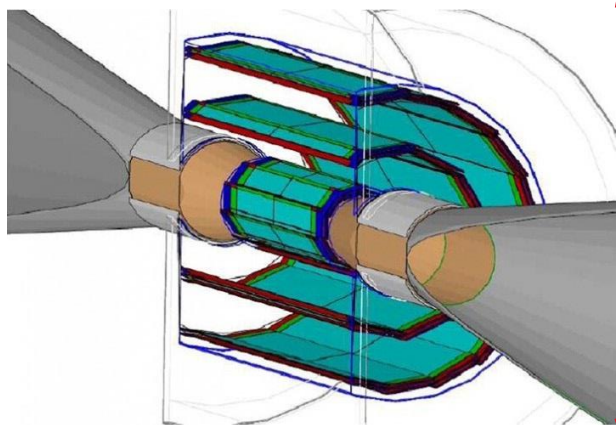
崩壊点検出器
