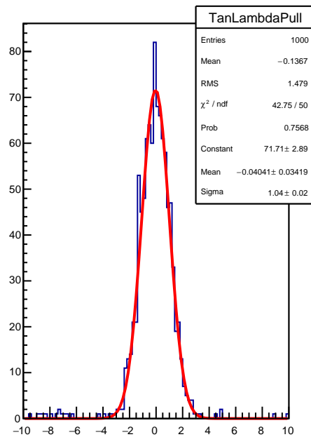
TanLambda
