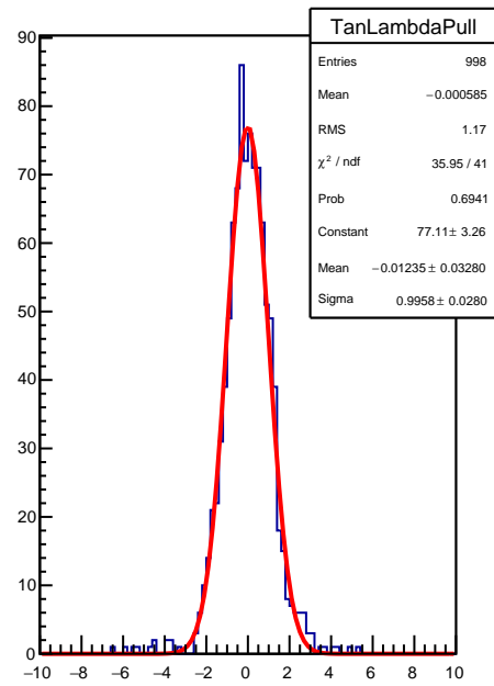
TanLambda
