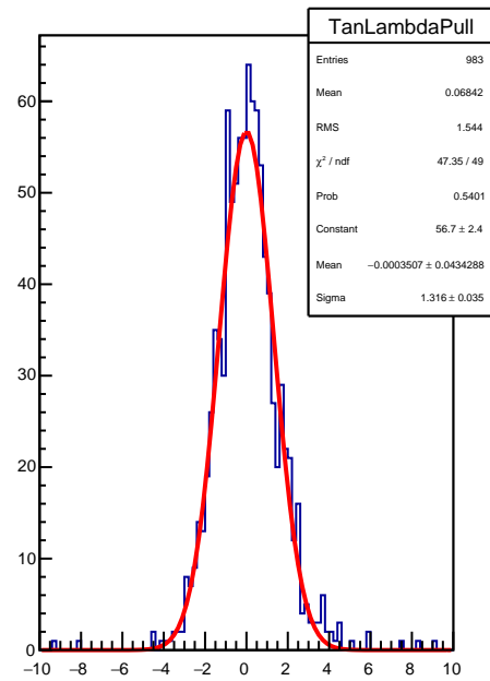
TanLambda
