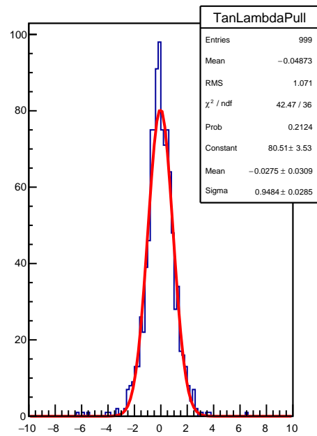
TanLambda
