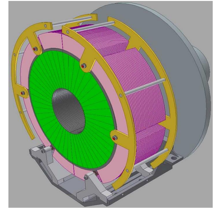
LumiCal
