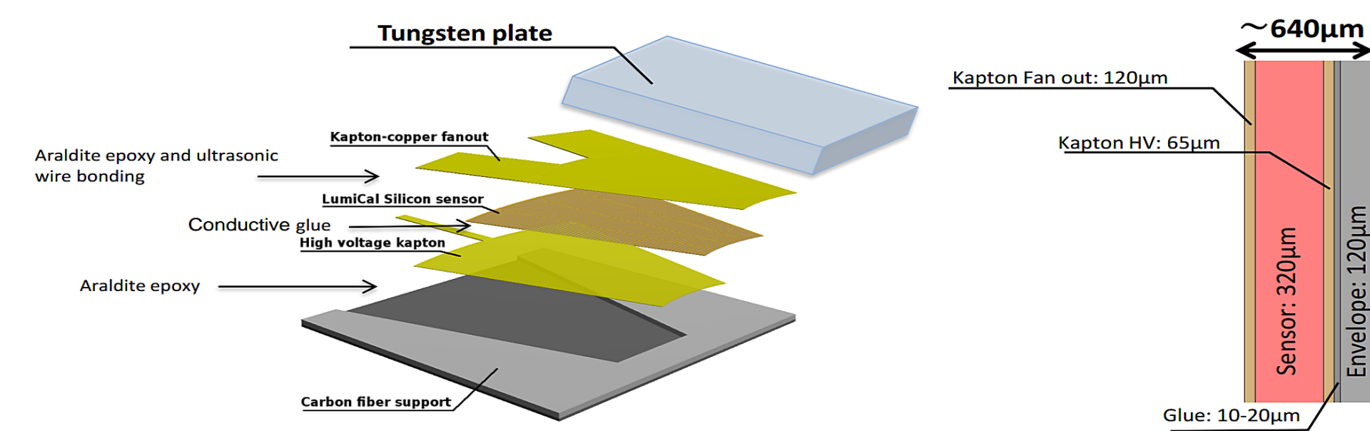
Thin LumiCal module
