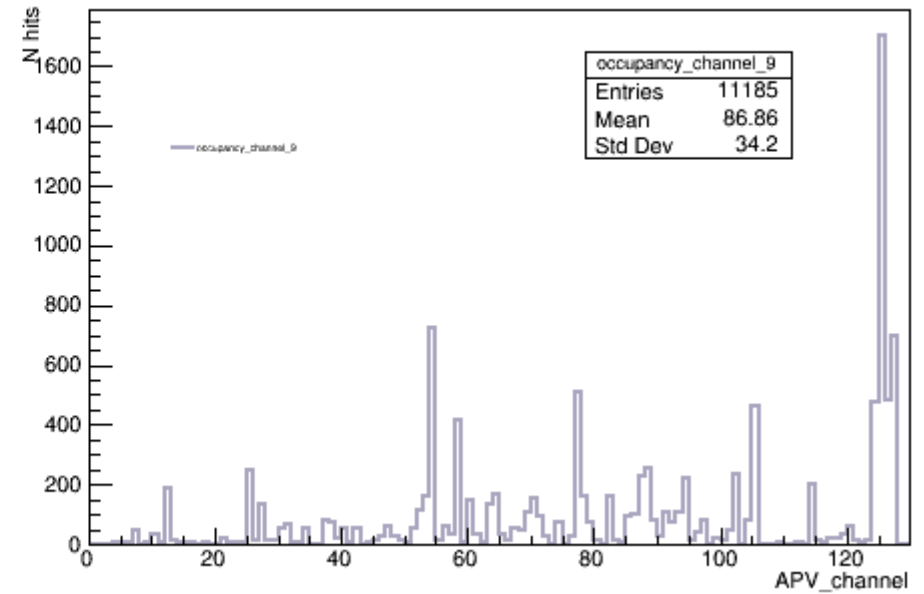
occupancy_channel_9
