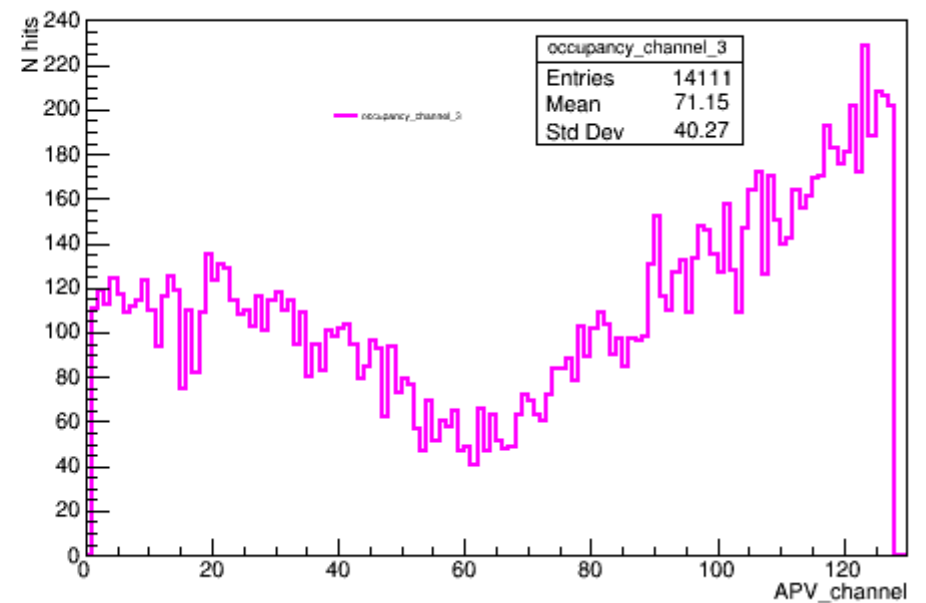
occupancy_channel_3
