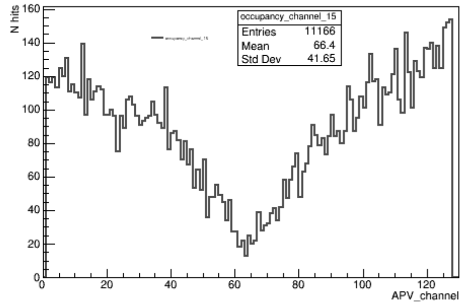
occupancy_channel_15
