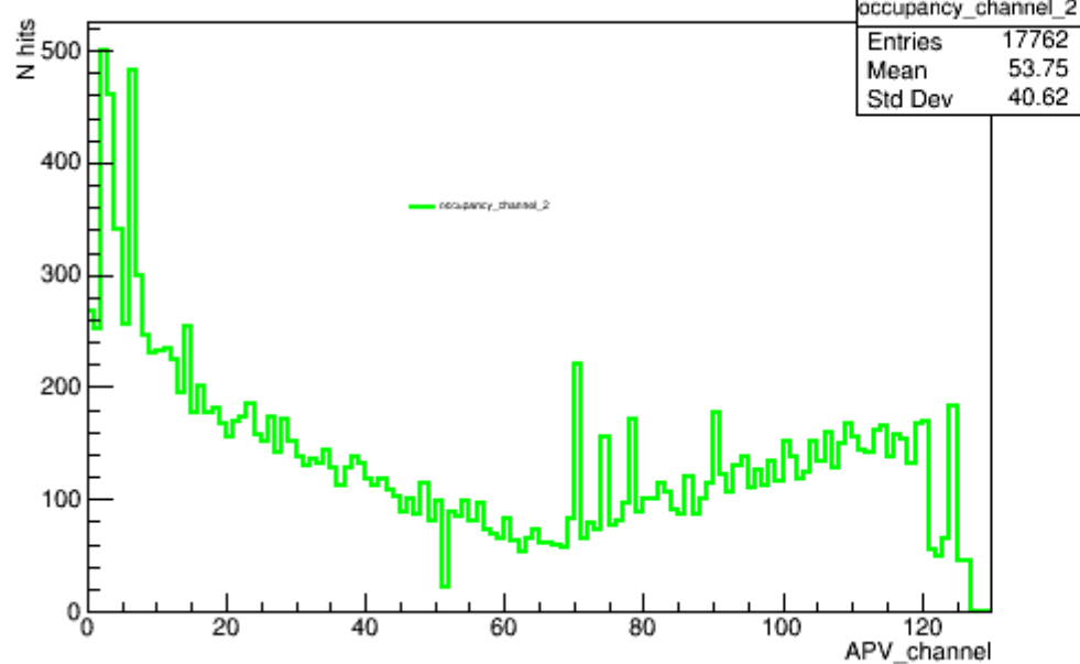
occupancy_channel_2
