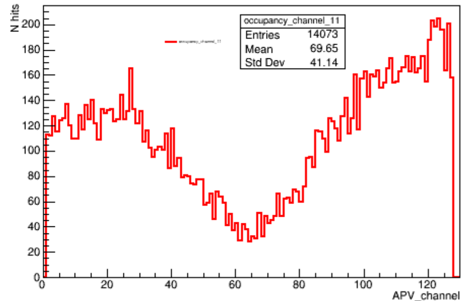
occupancy_channel_11
