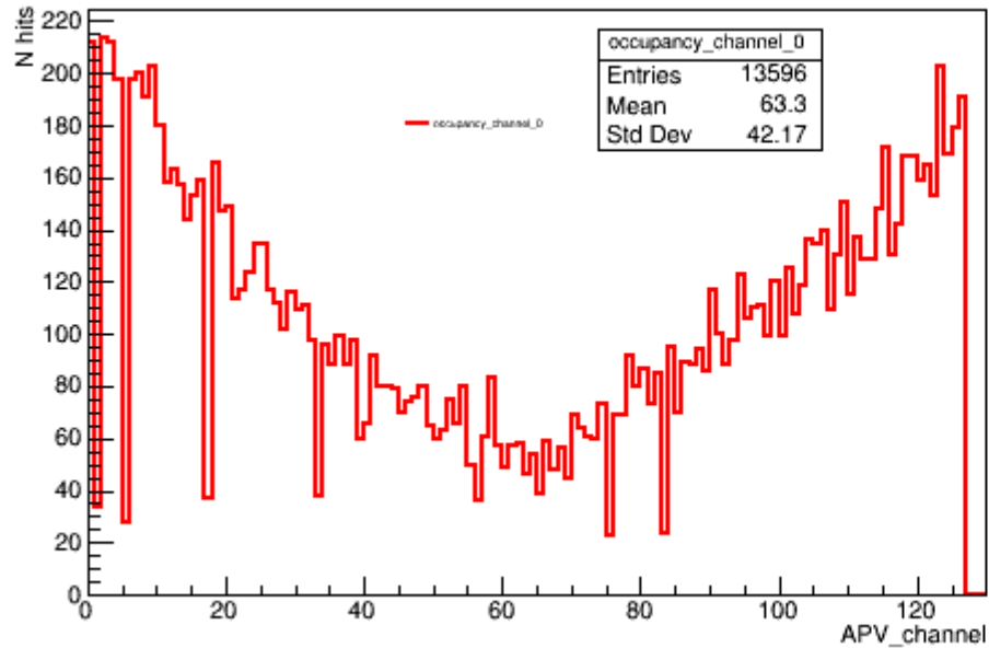
occupancy_channel_0
