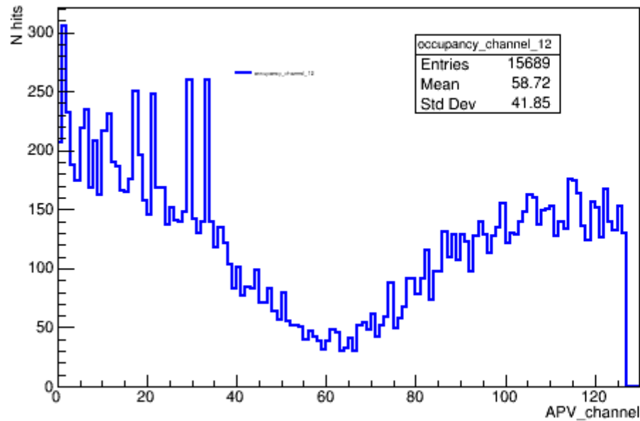
occupancy_channel_12
