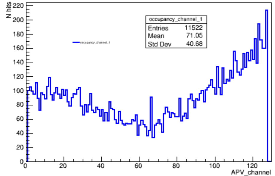
occupancy_channel_1
