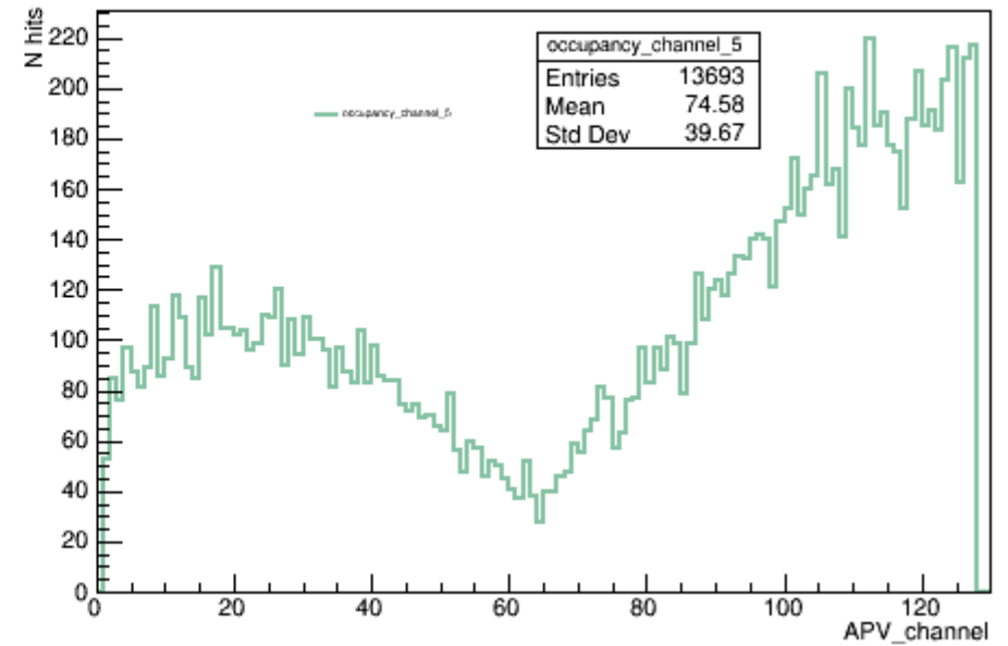
occupancy_channel_5
