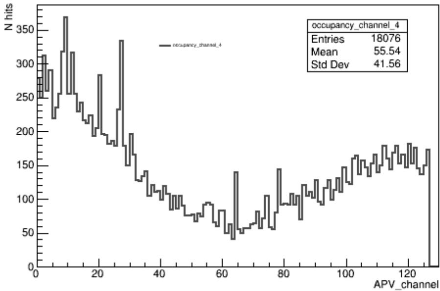
occupancy_channel_4
