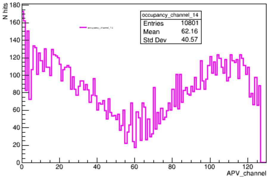
occupancy_channel_14
